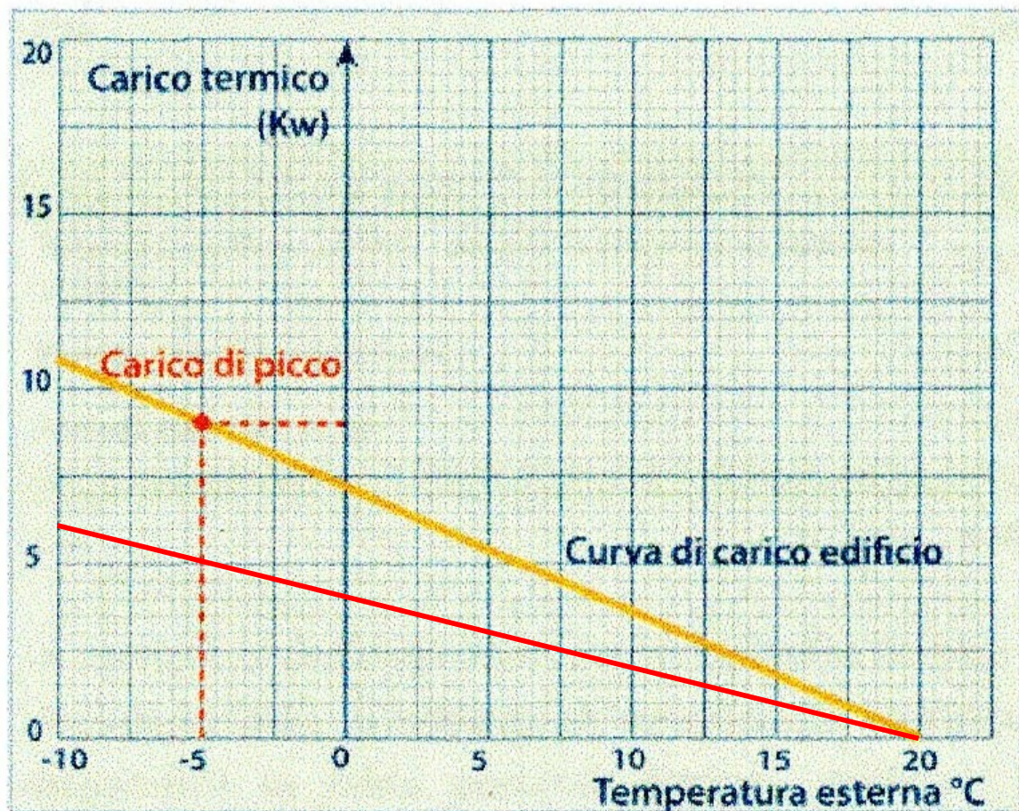
fig. 4.1 Curva di carico termico dell'edificio
